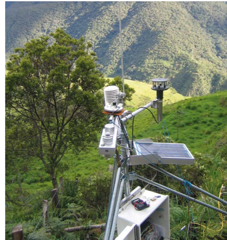
Die meteorologische Station am Rio San Francisco in Süd-ecuador wird seit 1997 betrieben. Sie steht in der Nähe der Forschungsstation Estación Científica San Francisco.
